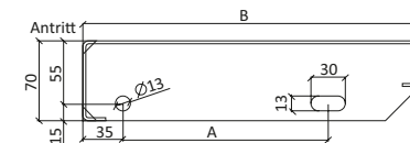
Bohrbild 1
